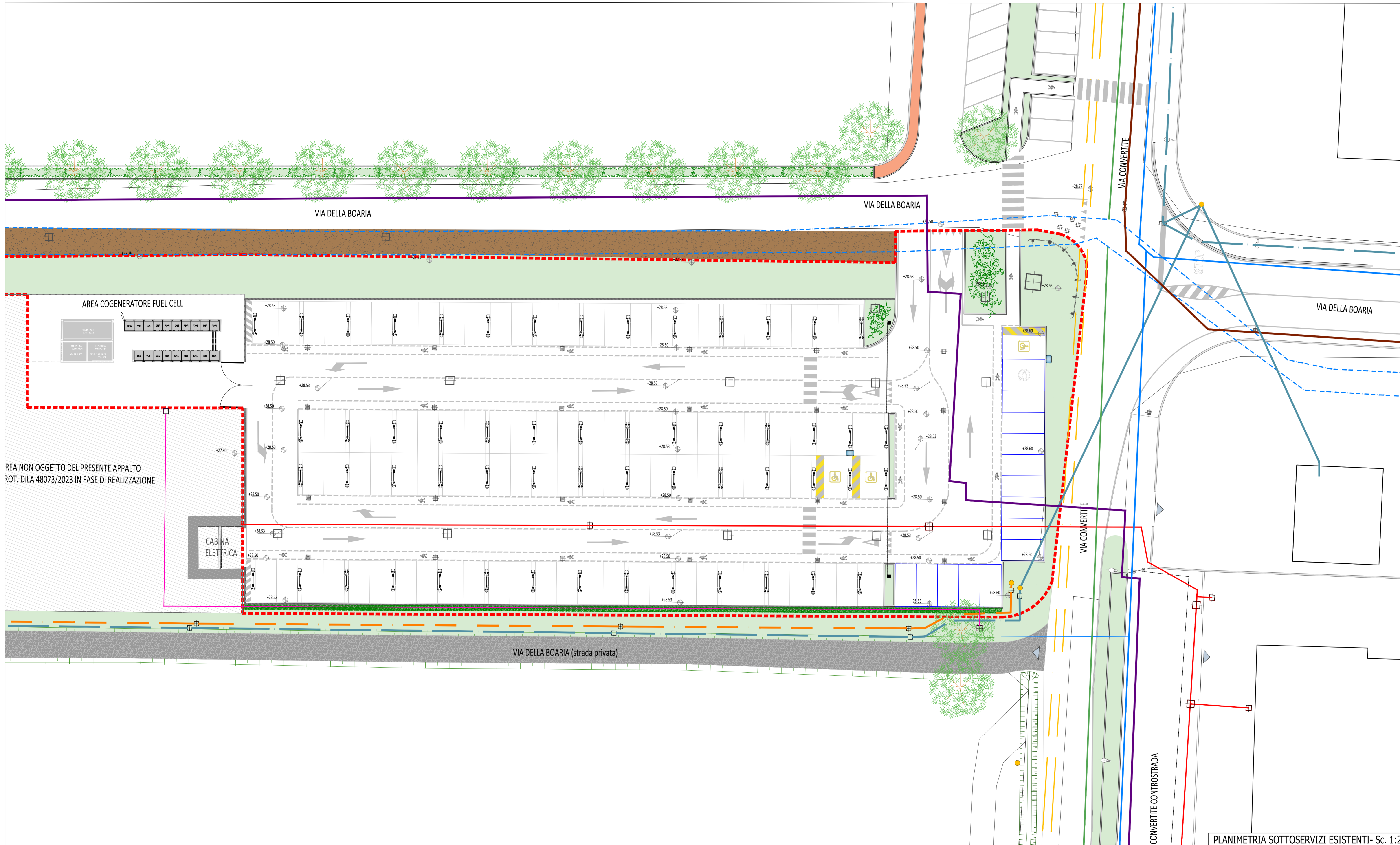
PLANIMETRIA SOTTOSERVIZI ESISTENTI- Sc. 1:200
